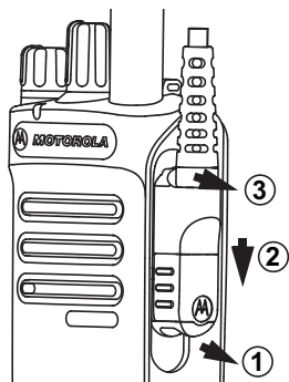
Figura 5: Colocar el conector de accesorios en el radio sin teclado
