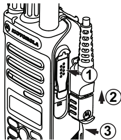
Figura 5: Fixar o conector do acessório ao rádio sem teclado
