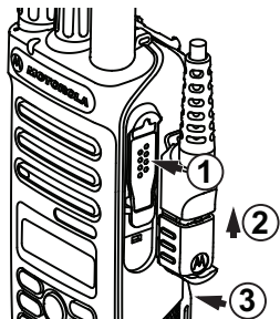
Figura 5: Colocar el conector de accesorios en el radio sin teclado
