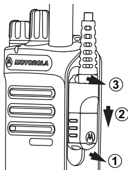
Figura 5: Fixar o conector do acessório ao rádio sem teclado
